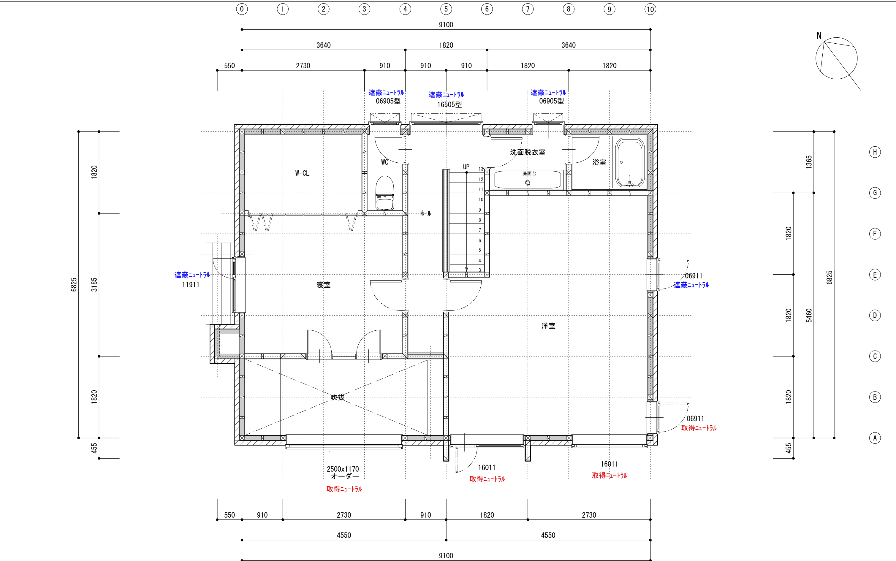
2階平面図 S=1/50
